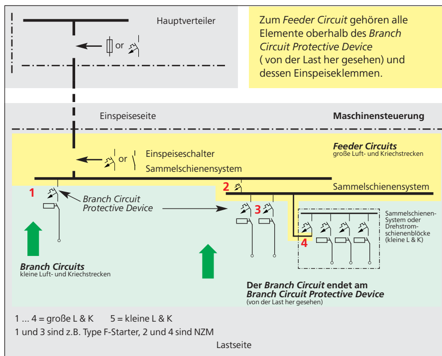
Bild 8: Das Bild zeigt zusätzlich eine Motorstarter-Gruppe. Das Sammelschienensystem oder die Drehstromschienenblöcke liegen im Branch Circuit , lediglich die Eingangsklemmen des Gruppen-Vorschaltenschutzorgans gehören zum Feeder Circuit . In diesem Fall reichen für das Sammelschienensystem und die Geräte (außer für die Eingangsklemmen des Vorschaltenschutzorgans) die kleinen Luft- und Kriechstrecken.
